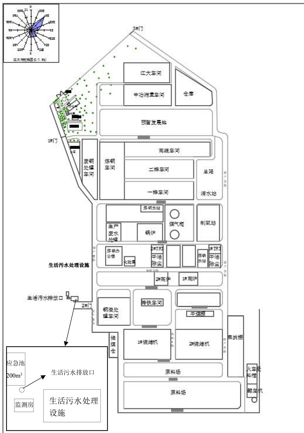
图 2.1-2 阳春新钢铁有限责任公司总平面布置图
