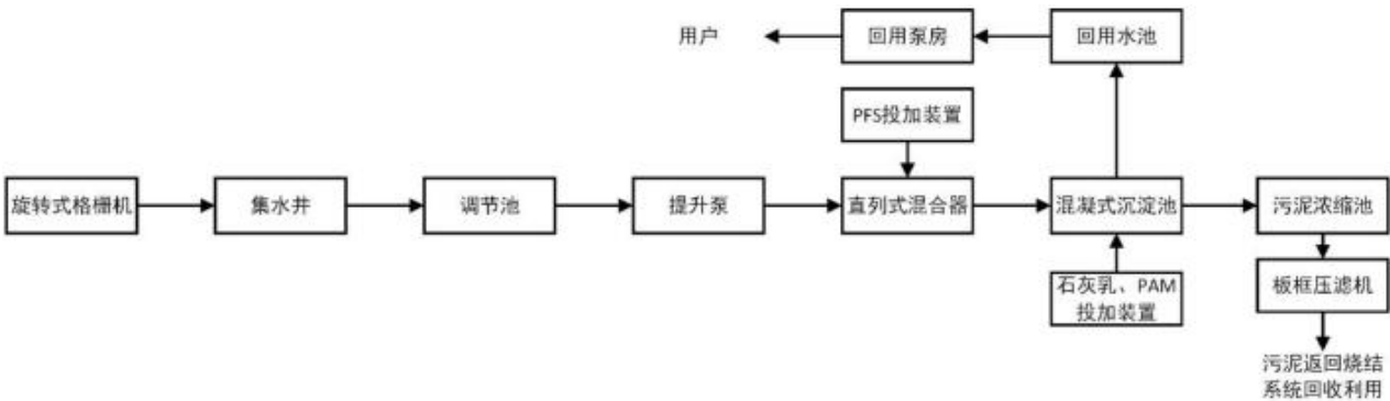
图 2.1-3 生产废水处理站工艺流程图
