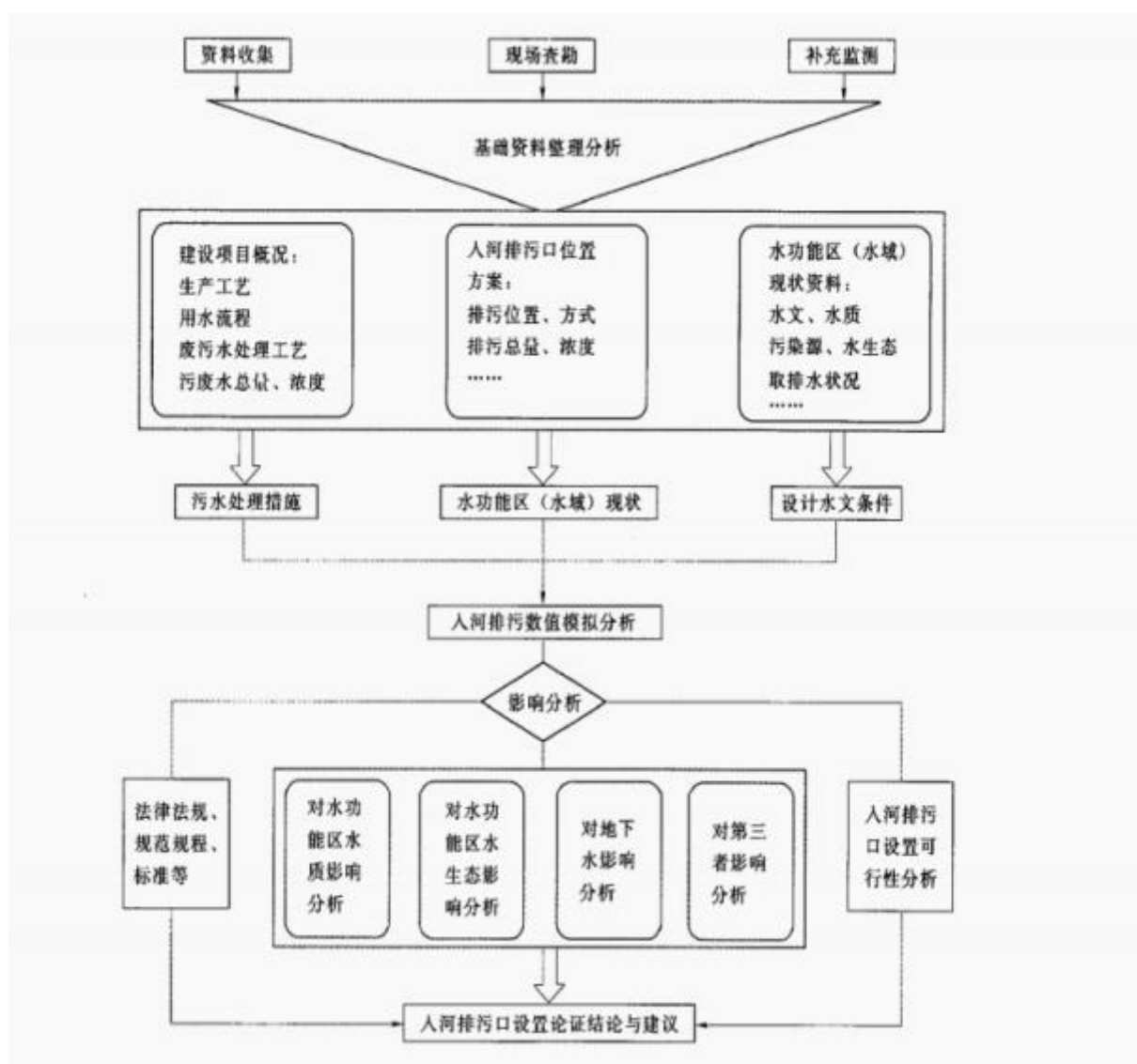
图 1.4-1 论证工作程序图
