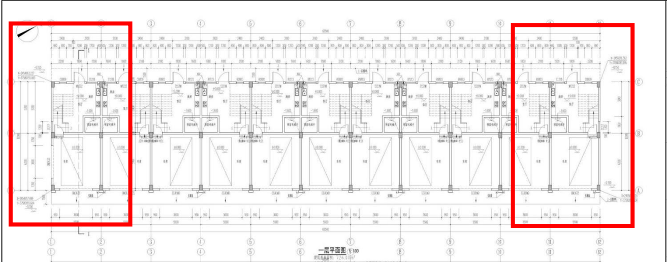
5 幢调整方案首层平面图
