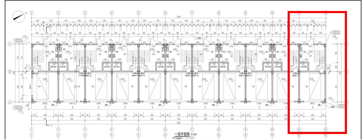
2 幢调整方案首层平面图
