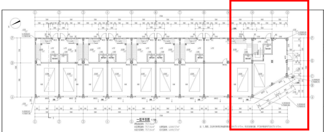
1 幢已批方案首层平面图
