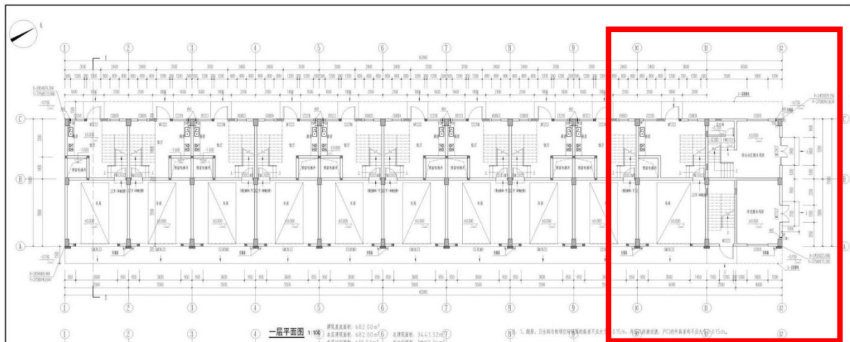
3 幢调整方案首层平面图
