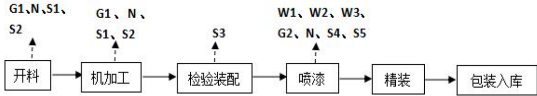
图 2-2 项目生产工艺流程图
