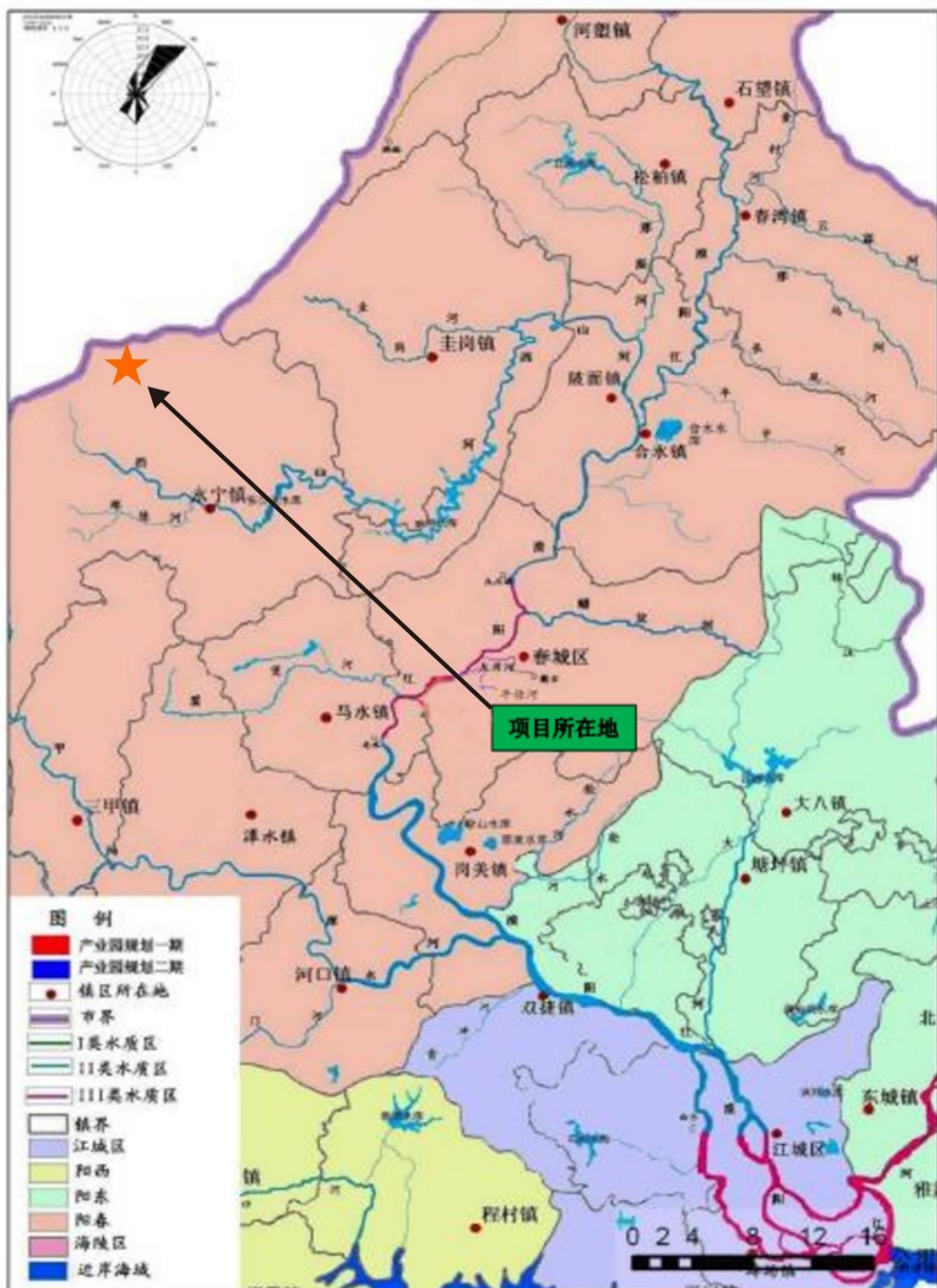
附图 5 建设项目水环境功能区划图
