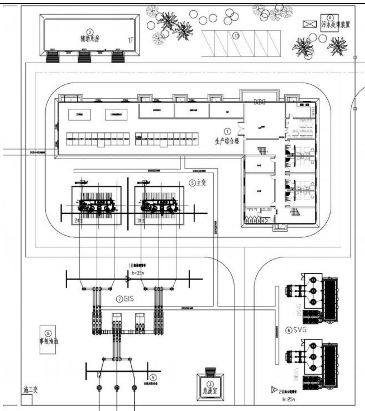
图 2-4 升压站平面布局示意图
