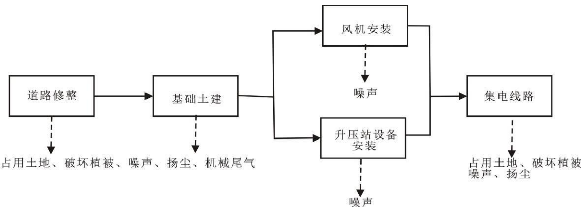
图 4-1 项目施工期污染环节示意图
