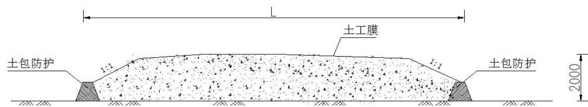
图 5-2 堆土区剖面图
