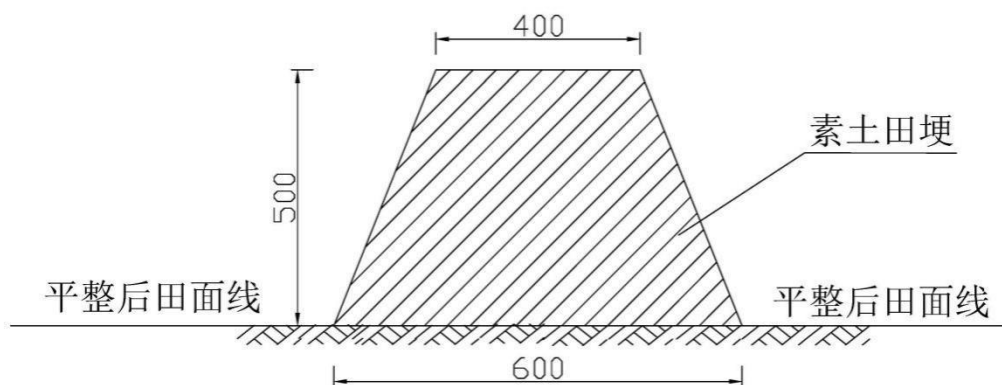
图8-2 田埂横断面设计示意图
