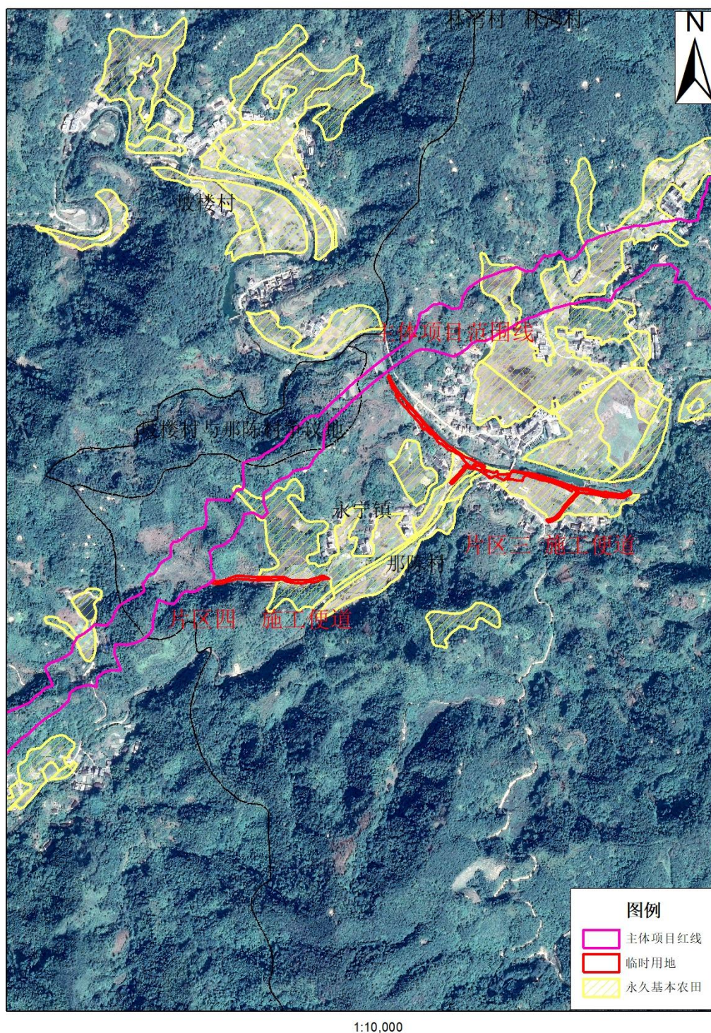
图3-1 片区三施工便道、片区四施工便道分布图
