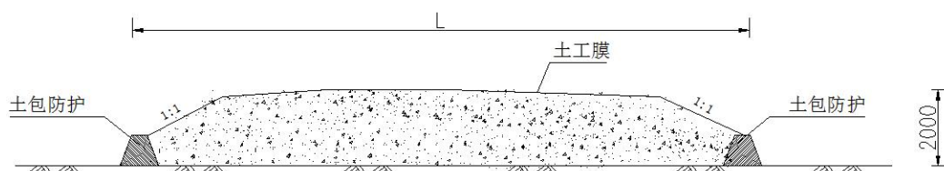
图 5-2 堆土区剖面图
