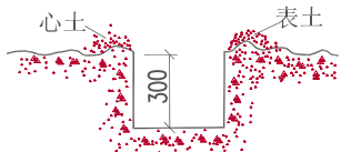
详图B 1:30
